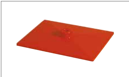
FUßPLATTE K Aus Kunststoff mit Rohraufnahme mittig Ø 12 mm, in OEK Standardfarben. Maße: 200x150 mm. Auch mit verzinkter Blecheinlage erhältlich. Fußplatte K | 20350-xx Mit Blecheinlage | 20351-xx
