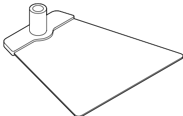
FUßPLATTE NT Trapezförmige Nirosta-Fußplatte aus nichtrostendem Edelstahl mit Rohraufnahme Ø 14 mm oder Ø 12 mm aus Kunststoff in OEK Standardfarben. Maße: 165(80)x160x1,5 mm Ø 14 mm | 20400-xx Ø 12 mm | 20401-xx
