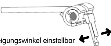
AUSFÜHRUNG „B“, für Haken mit untenliegendem Querdraht (z.B. Hohage, Wanzl und TEGO) 28718-00B
