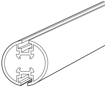
SYSTEMROHR QUICKPRICE QP Aluminium eloxiert, Rohr-Ø 25 mm, Standardlänge 200 cm. Sonderlackierungen auf Anfrage erhältlich. 15410-90/2000
