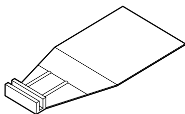
FUßPLATTE RS 200X90 Aus bruchsicherem Kunststoff zur direkten Aufnahme von Rahmen Reihe 100, grau. Andere Farben auf Anfrage erhältlich. Maße: 200x90 mm
