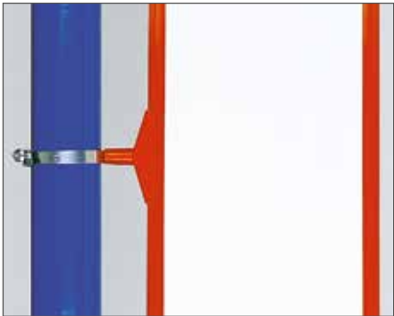
ROHRSCHELLE Zur Befestigung von Rahmen an Rohren mit Ø > 25 mm, Rohrschelle verzinkt und mit Schraube stufenlos feststellbar. T-Stück bitte separat bestellen. Ø 25-40 mm | 21740-00 Ø 40-60 mm | 21741-00 Ø 60-80 mm | 21742-00
