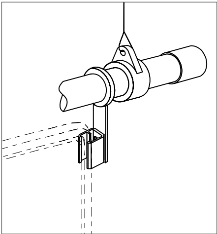
ENDKAPPE Passend zu Plakatschiene Rundrohr, für einen sauberen Schienenabschluß, grau 25170-03
